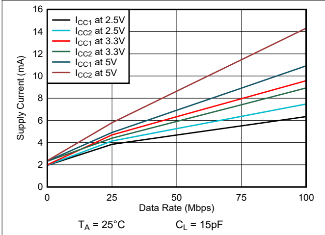
图 5-7. ISO7731 电源电流与数据速率间的关系 (具有 15pF 负载)
