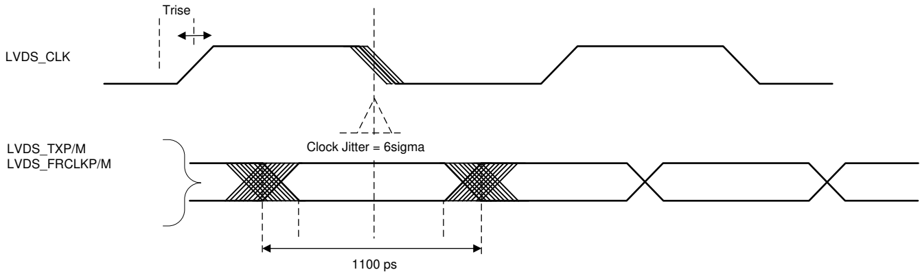
图 7-12. 计时参数
