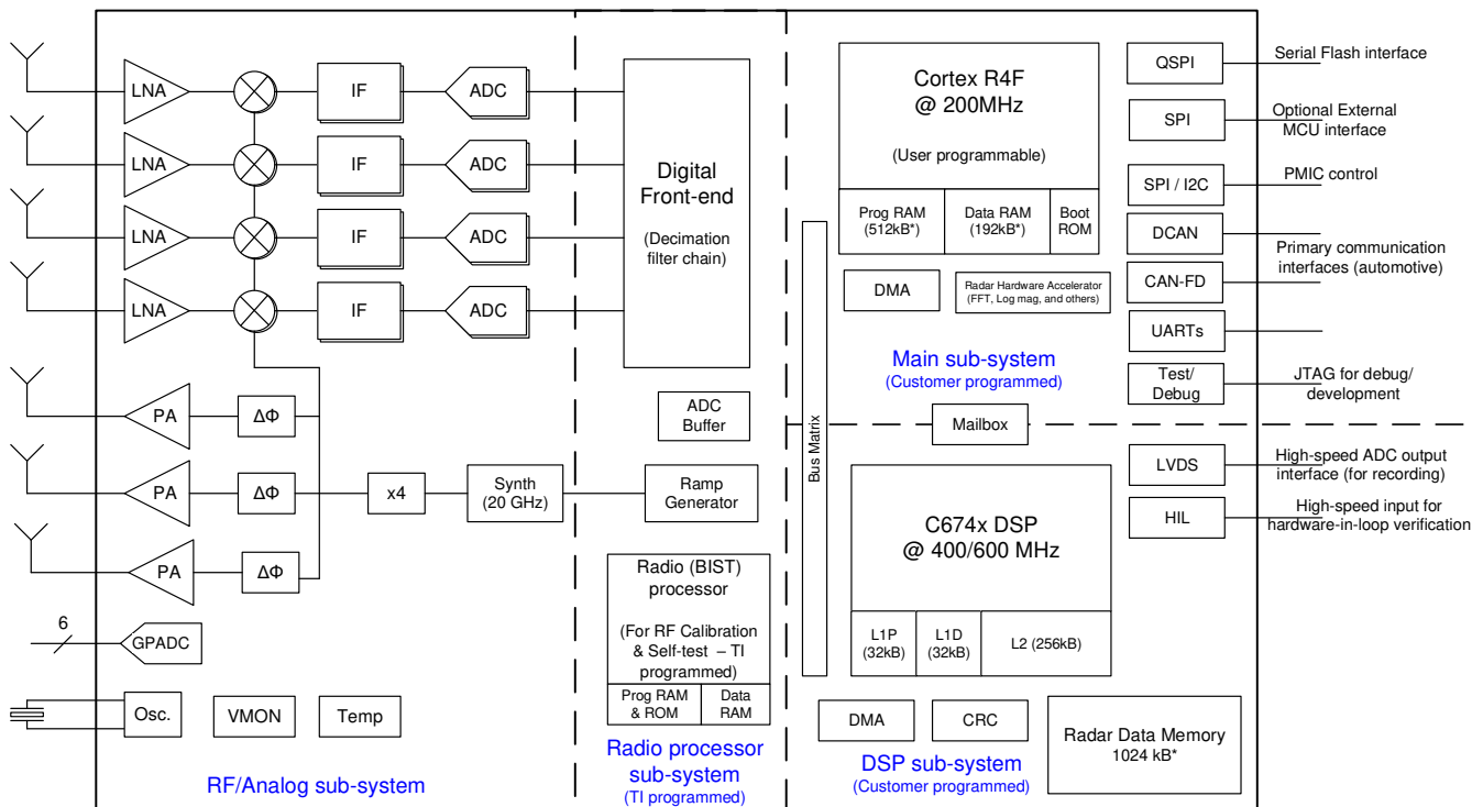
图 8-1. 功能方框图
