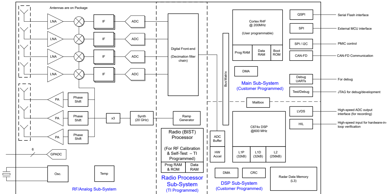
图 4-1. 功能方框图
