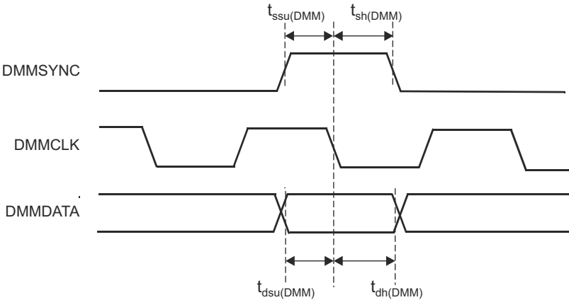
图 7-22. DMMDATA 时序
