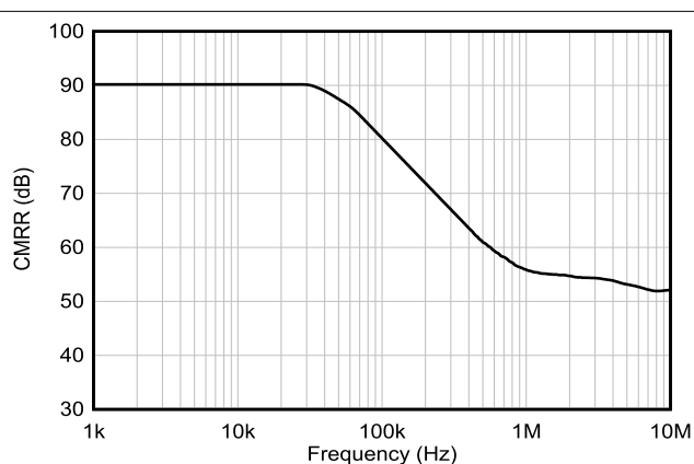
图 6-8. CMRR 与频率间的关系
