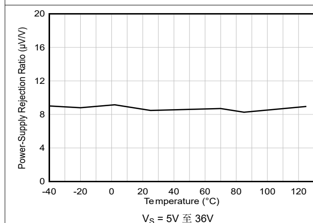
图 6-11. 电源抑制比与温度间的关系
