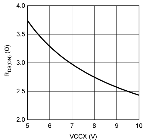
图 5-24. VCCX Switch R_{DS(ON)} vs VCCX
