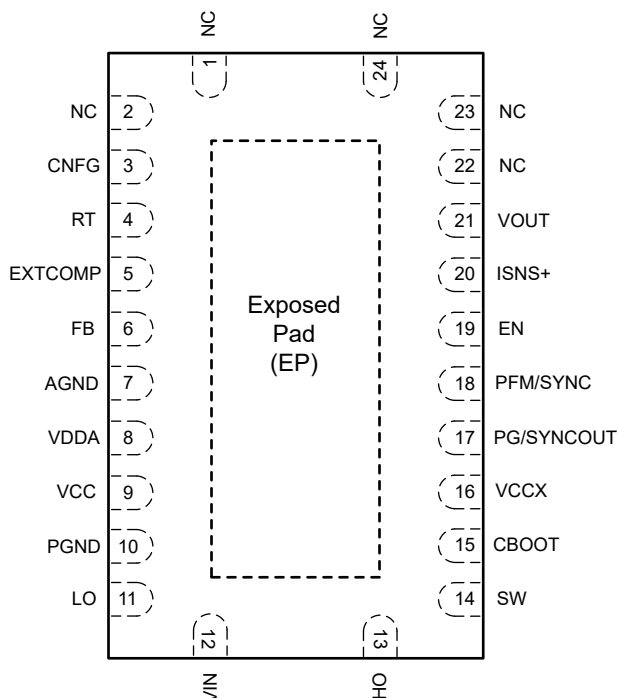
图 6-1. (Top View)
