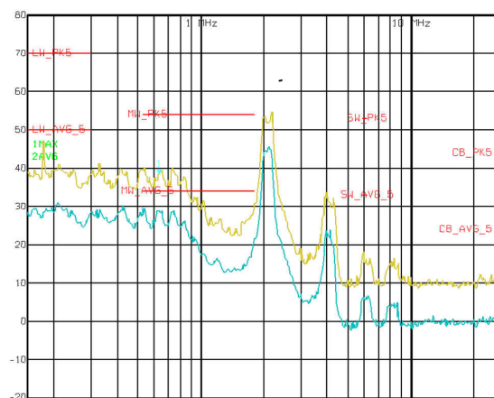
CISPR 25 EMI 性能, 150kHz 至 30MHz
