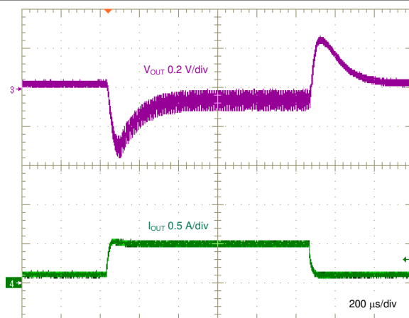
图 8-11. Load Transient, 0.1 A to 1 A, 0.1 A/μs
