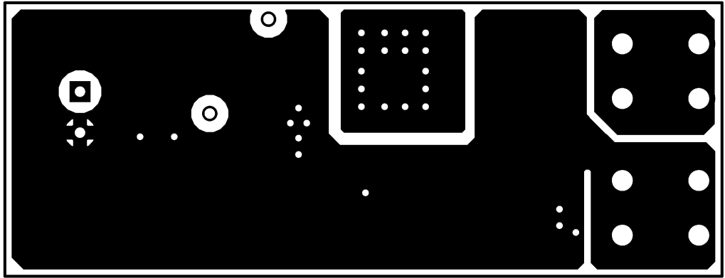
图 7-12. 焊接侧
