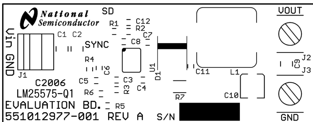
图 7-13. 丝印
