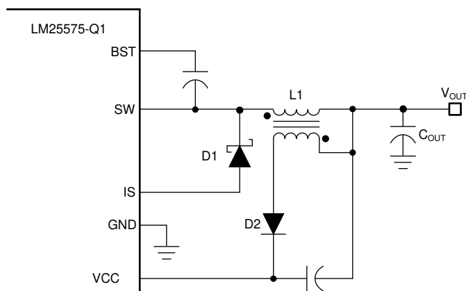
图 7-2. 输出电感器上带有额外绕组的 V_{CC} 偏置
