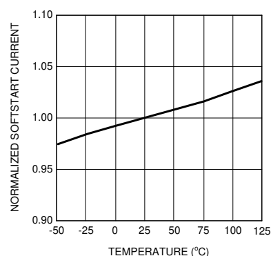
图 5-2. 软启动电流与温度间的关系
