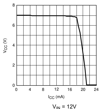
图 5-3. V_{CC} 与 I_{CC} 间的关系
