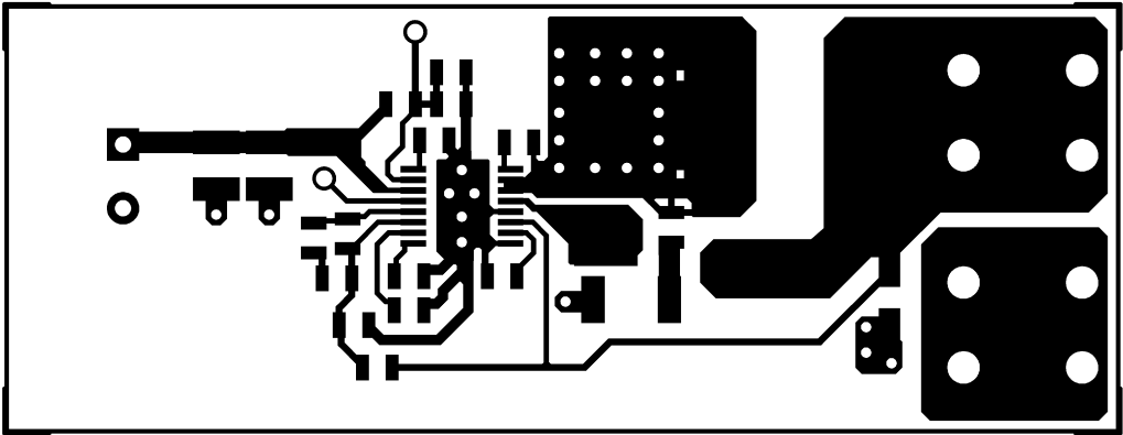
图 7-11. 组件侧
