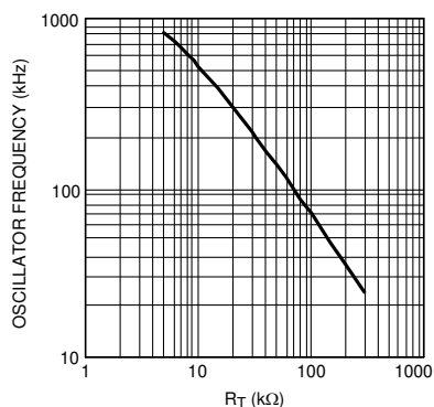
图 5-1. 振荡器频率与 R_T 间的关系
