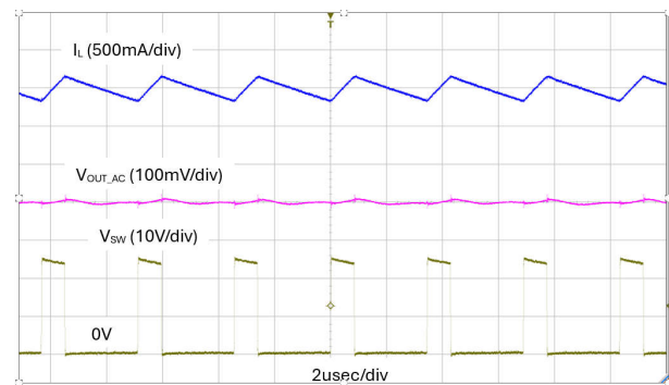
图 7-9. 稳态波形
