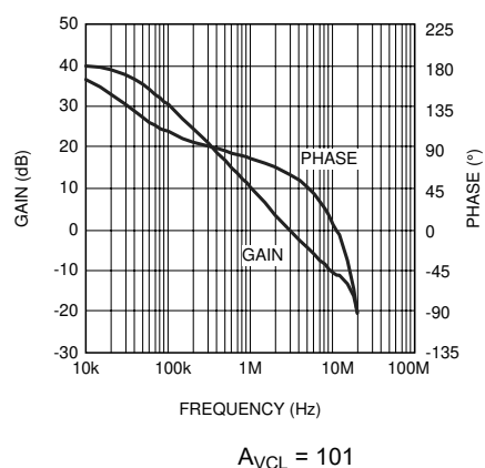
图 5-5. 误差放大器增益与相位
