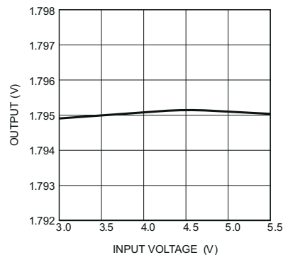
图 5-8. 线性调整率
