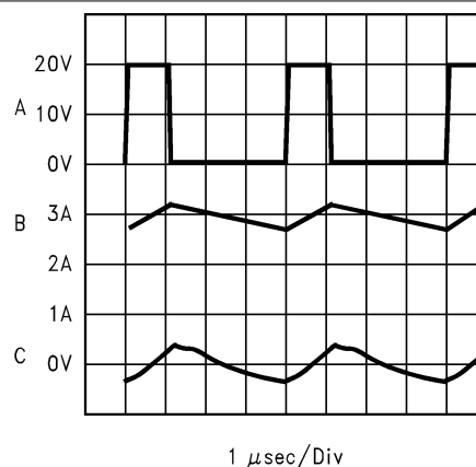
图 5-10. 开关频率
