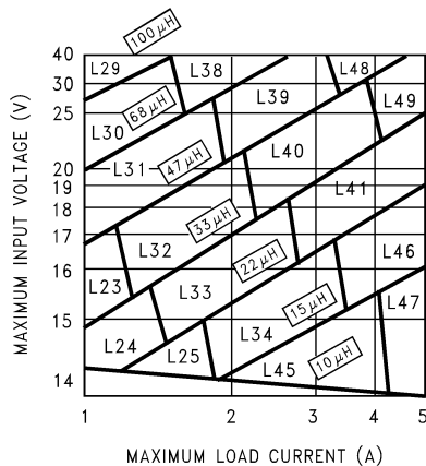
图 7-4. LM2678-12
