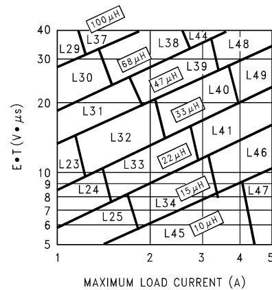
图 7-5. LM2678 可调节
