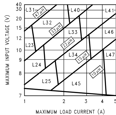
图 7-3. LM2678-5
