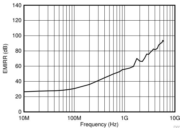
图 6-28. 以同相输入为基准的电磁干扰抑制比 (EMIRR+) 与频率间的关系 D035
