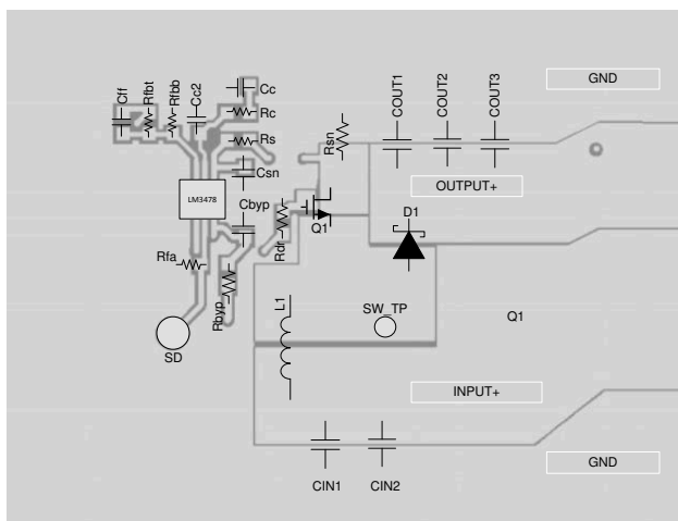
图 7-12. 升压转换器的典型布局
