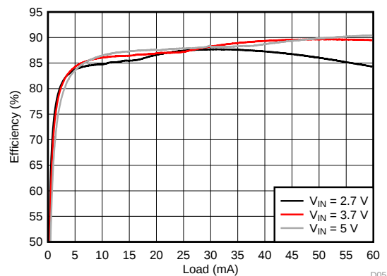
背光效率, 2P8S
