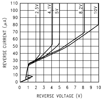
图 5-3. 反向特性和最小工作电流
