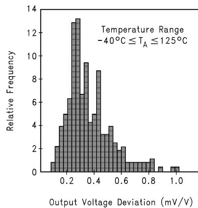
图 5-5. 热迟滞
