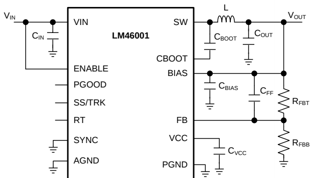
简化原理图
