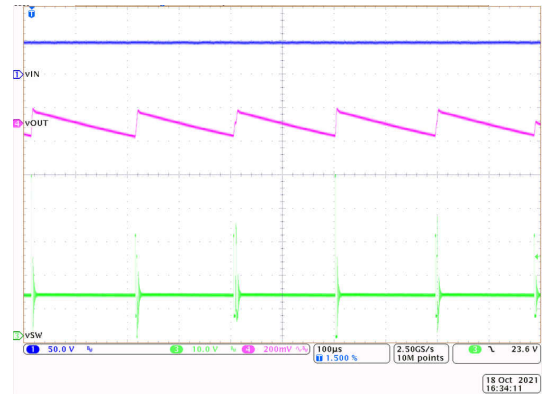
图 8-9. Light-Load Switching
