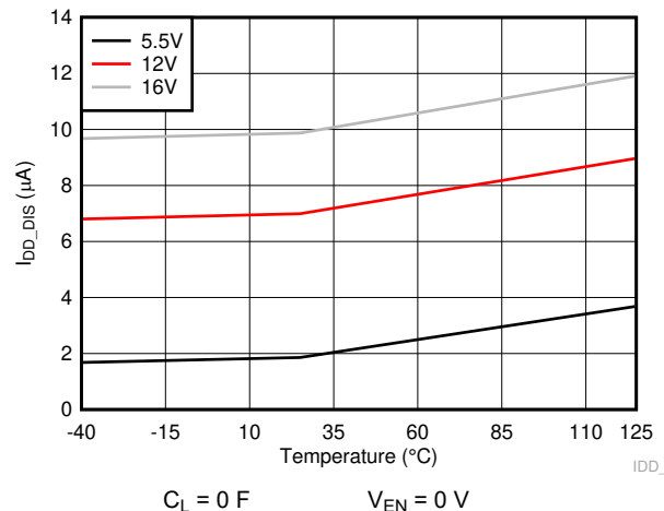
图 6-6. VDD Current When Disabled
