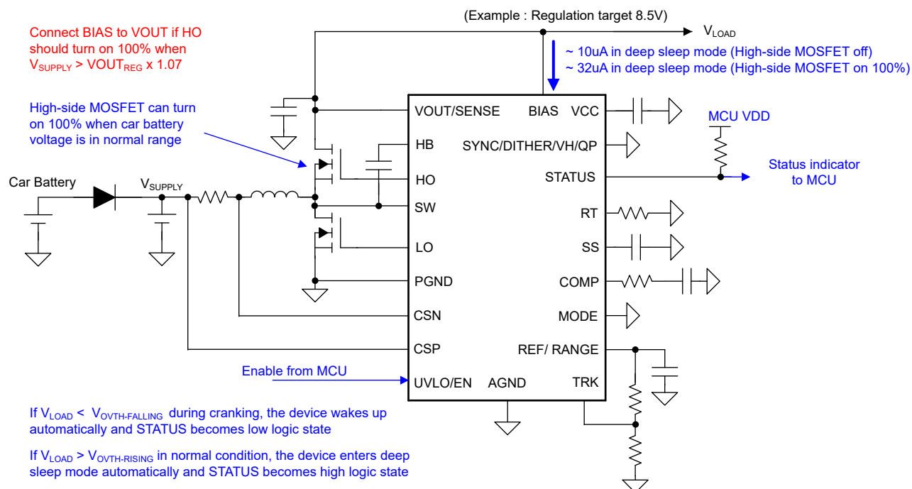
图 10-7. LM5152-Q1 在汽车预升压应用
