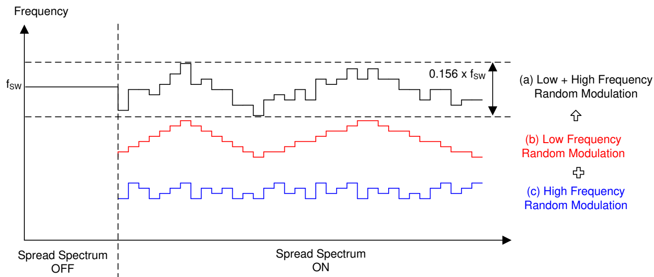
图 8-9. Dual Random Spread Spectrum
