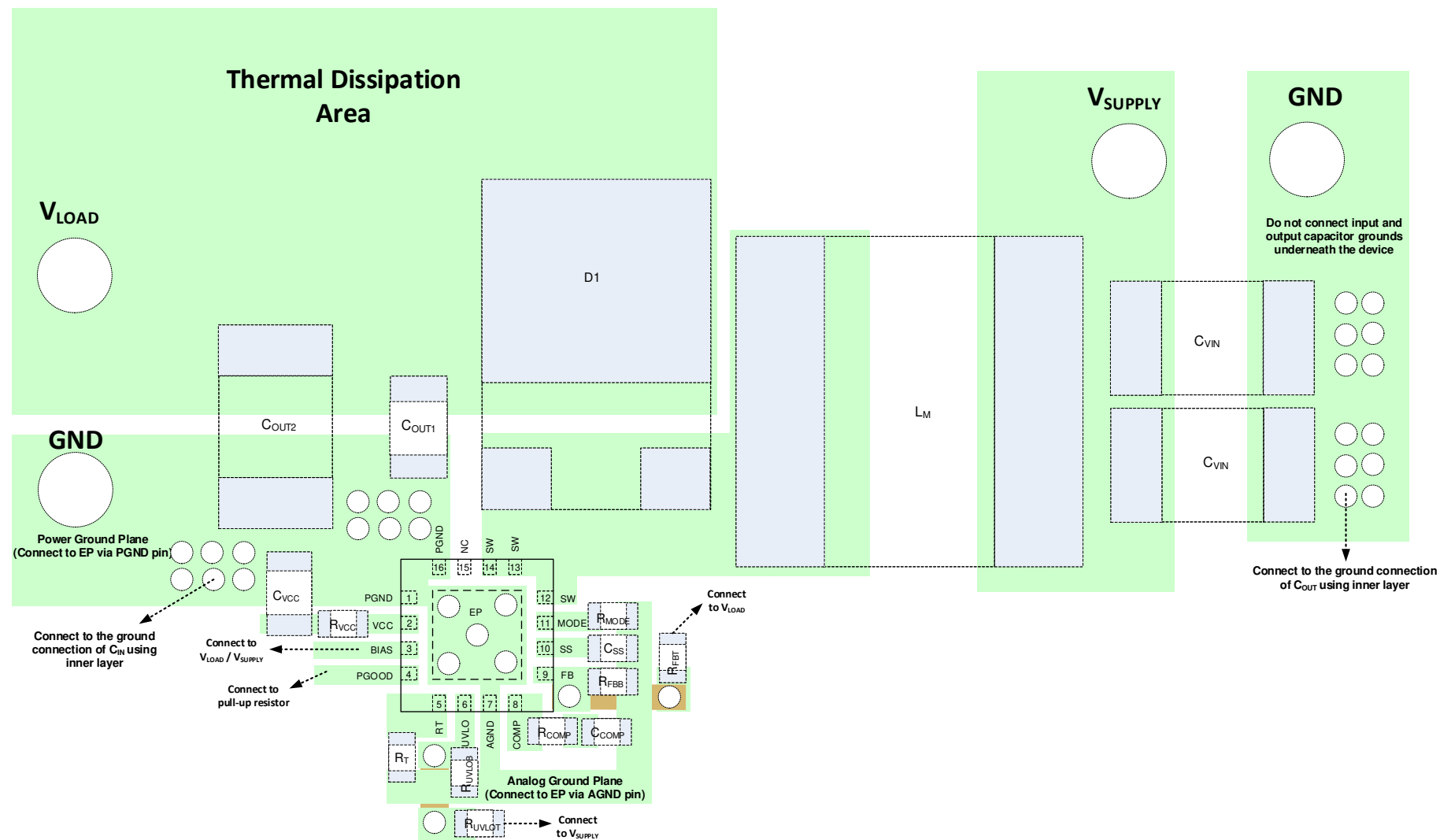
图 11-1. PCB Layout Example
