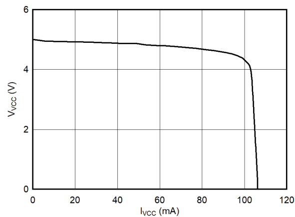
图 7-5. V_{VCC} vs I_{VCC}
