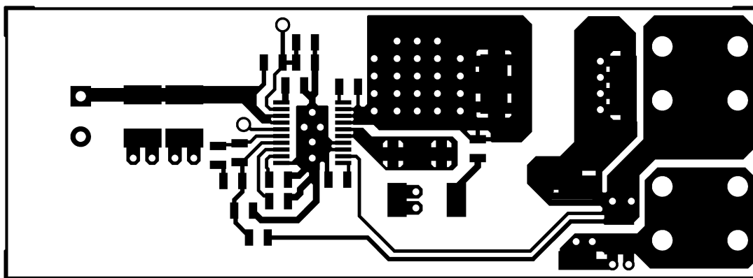
图 7-14. 组件侧
