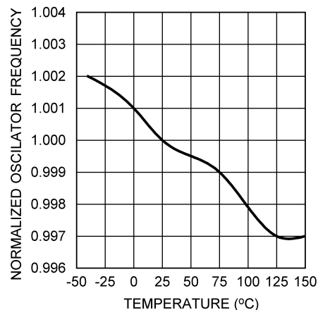
图 5-2. 振荡器频率与温度间的关系 (Q0) F_{osc} = 200\text{kHz}
