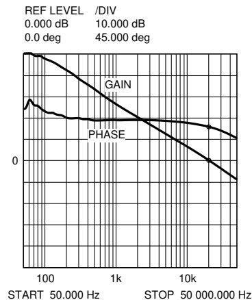
图 7-12. 总体环路增益与相位
