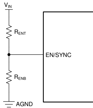
图 9-3. UVLO Using EN
