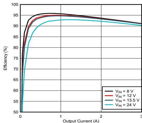
图 9-5. LM61430-Q1 Efficiency
