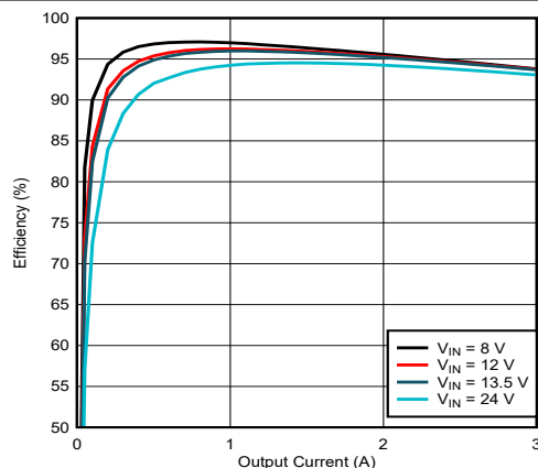
图 9-7. LM61430-Q1 Efficiency
