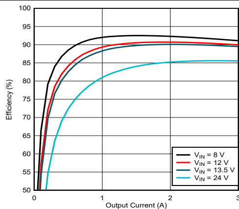
图 9-5. LM61430-Q1 Efficiency
