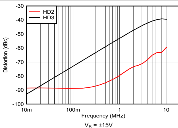
图 5-36. 谐波失真与频率间的关系
