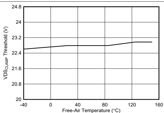
图 6-11. VDS_CLAMP Threshold vs Temperature
