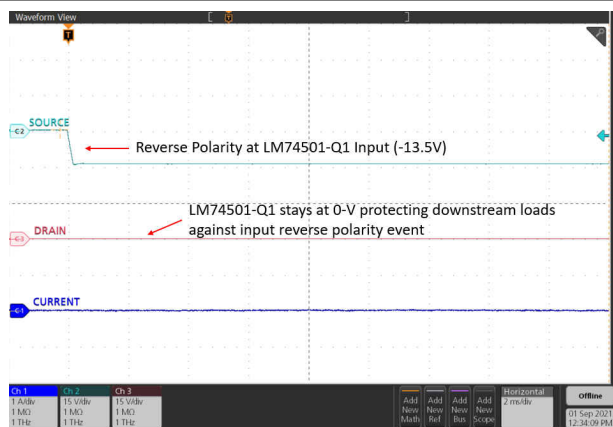
图 9-10. Input Reverse Polarity Hot Plug
