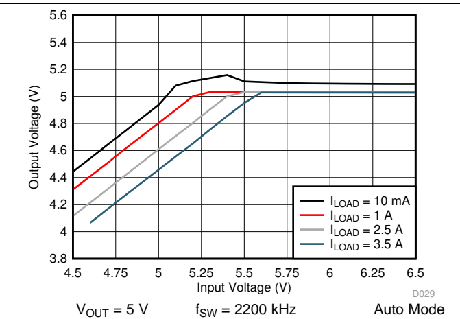
图 54. LM76003-Q1 Dropout Curve
