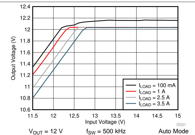
图 56. LM76003-Q1 Dropout Curve
