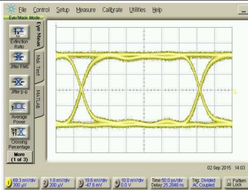
图 1. 75 Ω OUT0 PRBS10 at 2.97 Gbps
