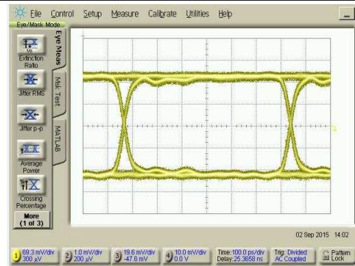
图 2. 75 Ω OUT0 PRBS10 at 1.485 Gbps
