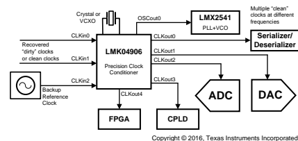
简化 LMK04906 方框图
