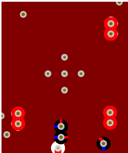
图 10-7. Recommended PCB Layout Bottom Layer
