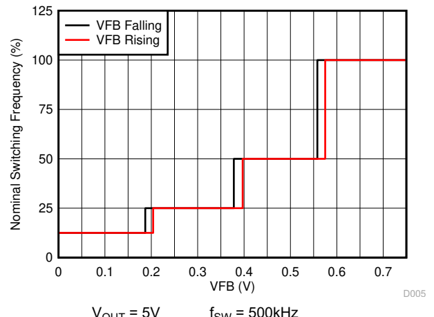
图 5-6. 频率与 V_{FB} 间的关系
