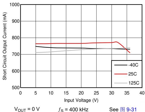
图 7-3. Short-Circuit Output Current
