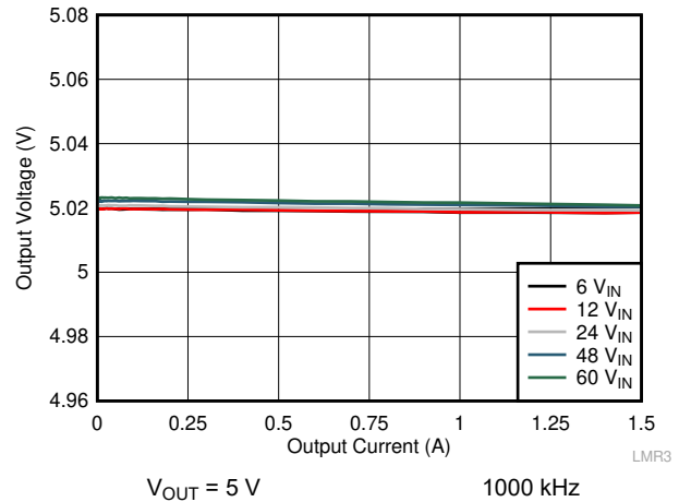
图 10-29. Load Regulation
