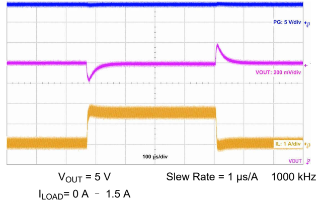
图 10-35. Load Transient
