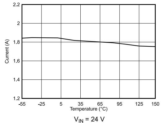
图 8-4. Low Side Current Limit
