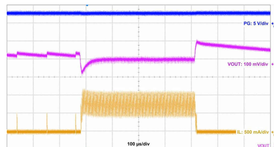
图 10-17. Load Transient
