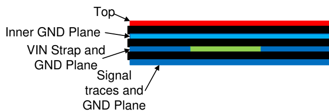
图 12-2. Example Layout
