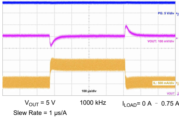
图 10-34. Load Transient
