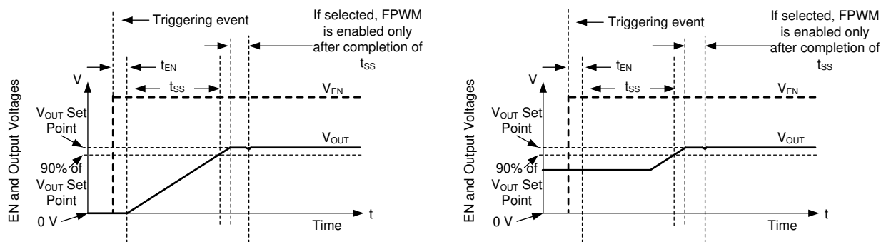
图 7-7. 带和不带预偏置电压的软启动/停止
