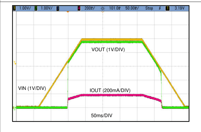
图 6-6. V_{OUT} = 5\text{V} 时的典型启动和关断
