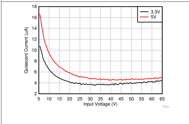
图 6-5. 输出电压固定为 3.3V 和 5V 且空载时的典型输入电源电流
