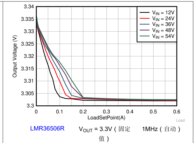
图 8-5. 线性和负载调整率
