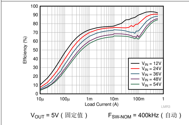
图 6-3. 5V 输出效率，自动模式
