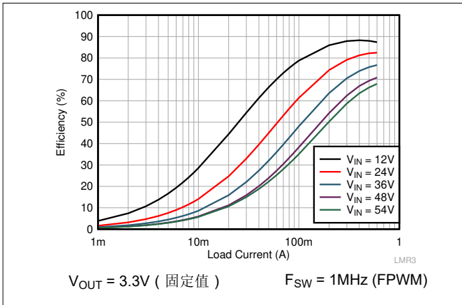
图 6-1. 3.3V 输出效率，FPWM
