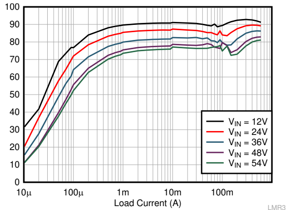
LMR36506R5 V_{OUT} = 5V (固定值) 1MHz (自动值)
