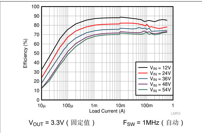
图 6-2. 3.3V 输出效率，自动模式
