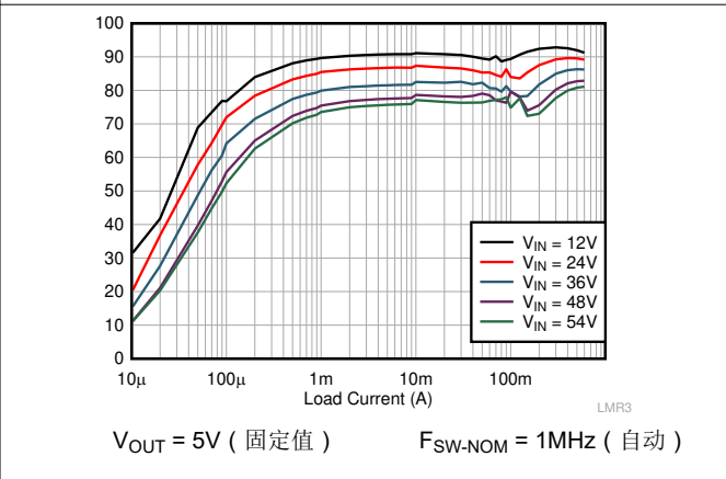
图 6-4. 5V 输出效率，自动模式
