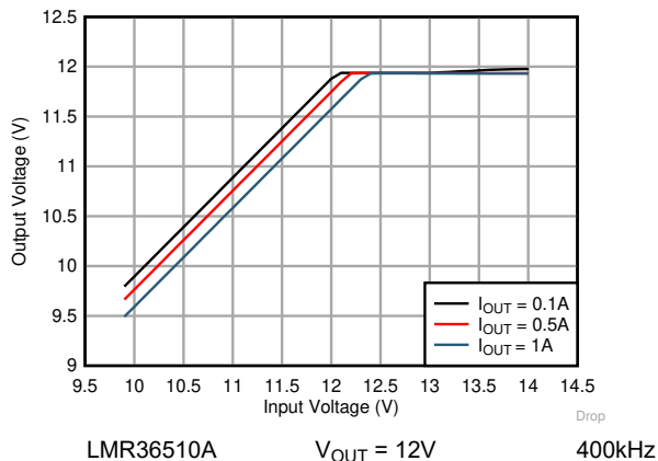
图 8-11. 压降特性
