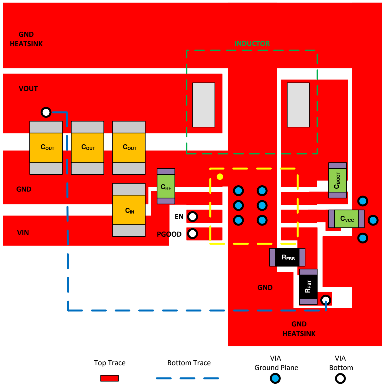
图 8-24. 示例布局
