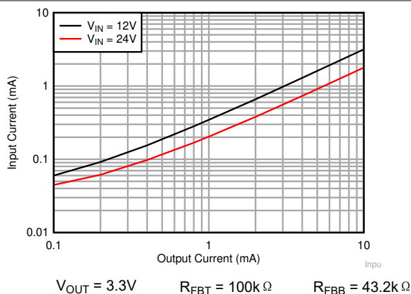
图 8-13. 输入电源电流与负载电流间的关系
