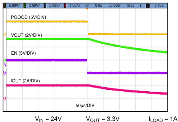
图 8-15. 使能关断波形
