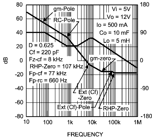
图 7：采用外部补偿的 LMR62421
