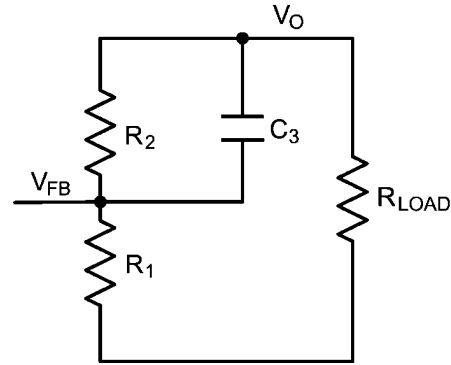
图 5: 设定 V_{OUT}
