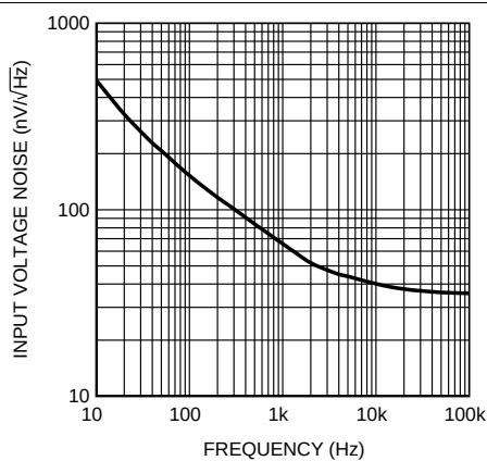
Figure 12. 输入电压噪声与频率间的关系
