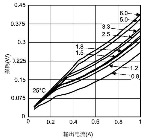
在25°C时12V输入效率
