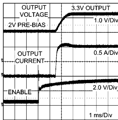
预偏置启动
