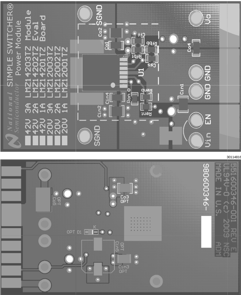
图1.评估印刷电路板顶部和底部视图
