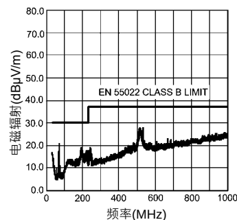
评估板电磁辐射值 (EN 55022 B级)
