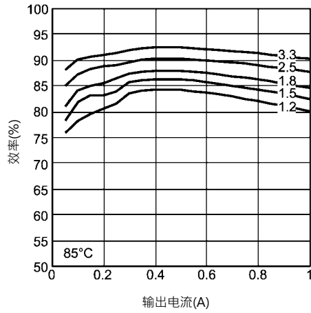
在85°C时6V输入效率
