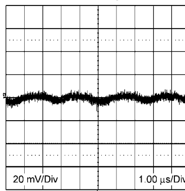
输出纹波 12V IN 3.3V O 1A
