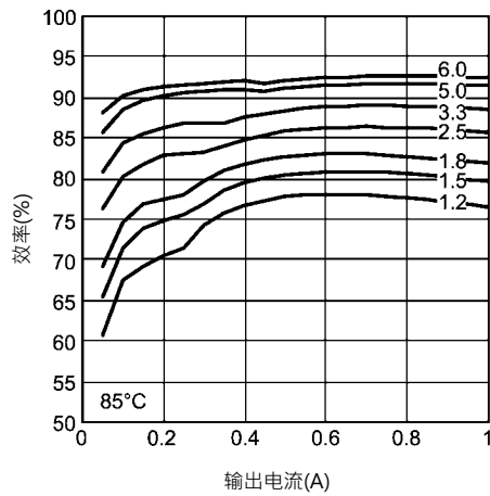
在85°C时12V输入效率
