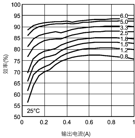
在25°C时12V输入效率
