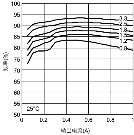
在25°C时6V输入效率
