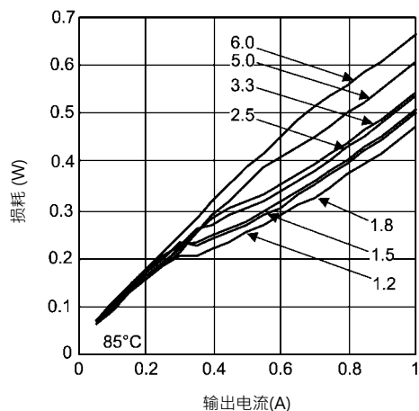
在85°C时20V输入消耗
