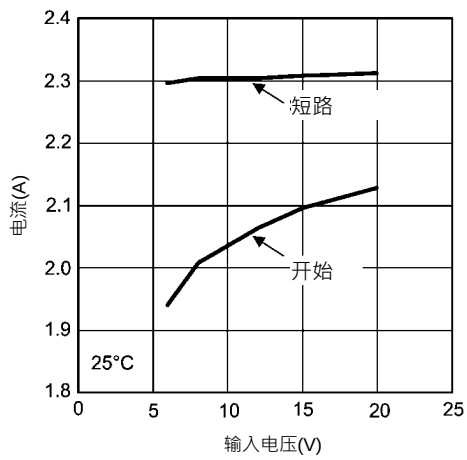
电流限制3.3V OUT @25°C
