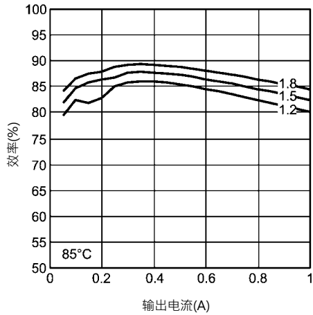
在85°C时5V输入效率
