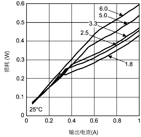
在25°C时20V输入消耗
