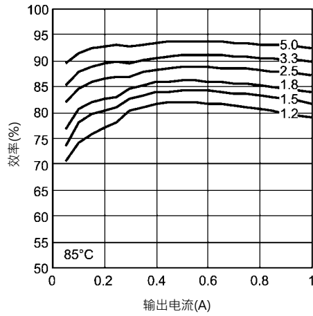
在85°C时8V输入效率
