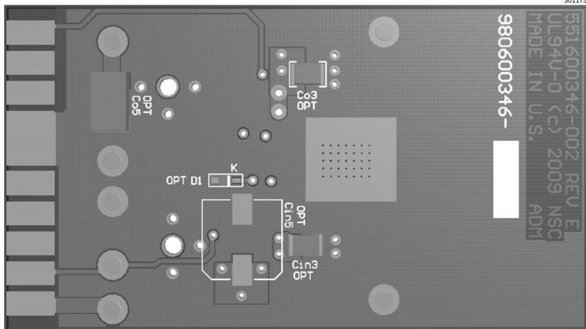
图1.评估印刷电路板顶部和底部视图
