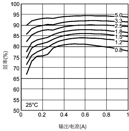
在25°C时8V输入效率
