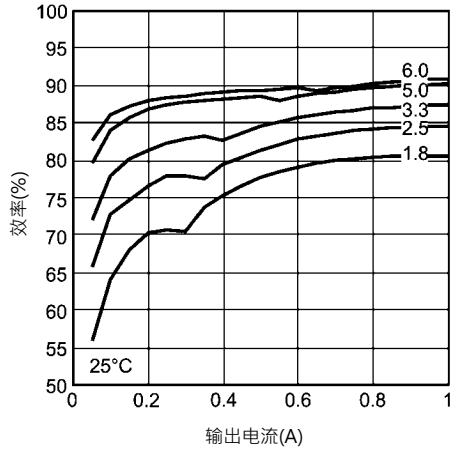
在25°C时20V输入效率
