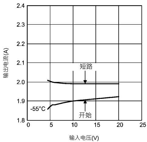
电流限制1.8V OUT @-55°C
