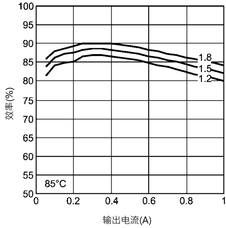
在85°C时4.5V输入效率
