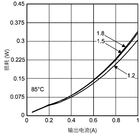
在85°C时4.5V输入消耗
