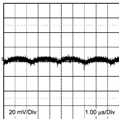
输出纹波
