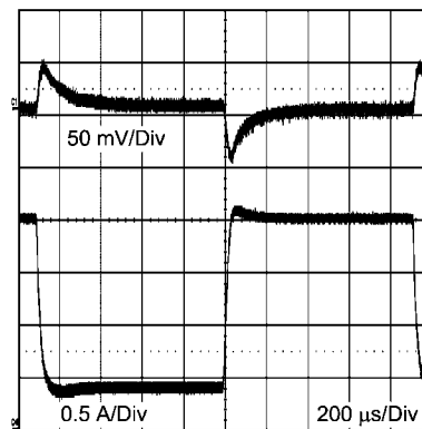
瞬态响应
