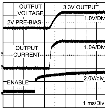
预偏置启动
