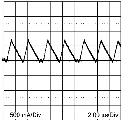
过渡模式运行 V_{IN} = 12V , V_O = 3.3V , I_O = 0.29A 2 \mu sec/div
