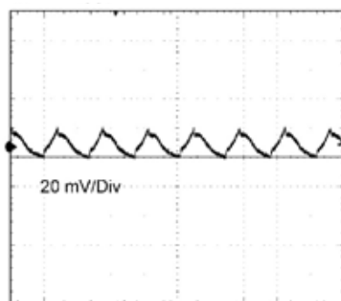
输出纹波 12 V IN , 3.3 V OUT (在满负载, 带宽 = 20 MHz)
