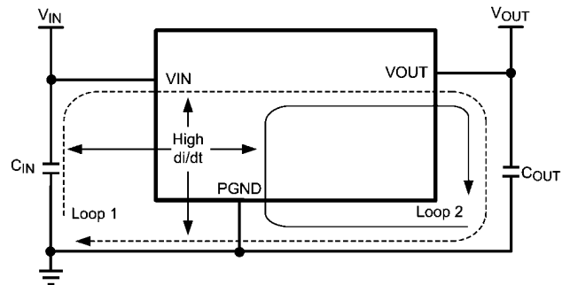
图3高电流回路
