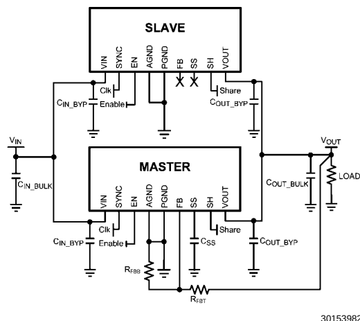
图4. 均流示例图
