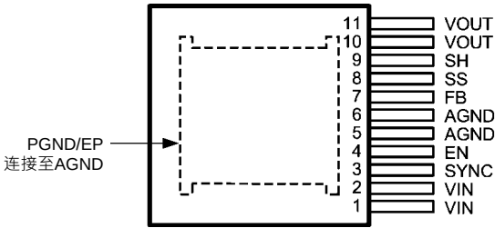
顶视图
