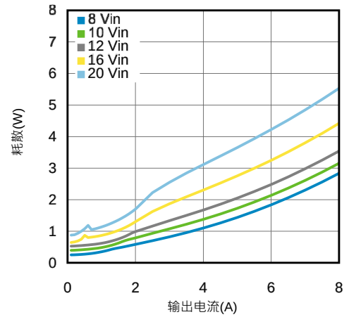
在25°C时5.0V输出耗散
