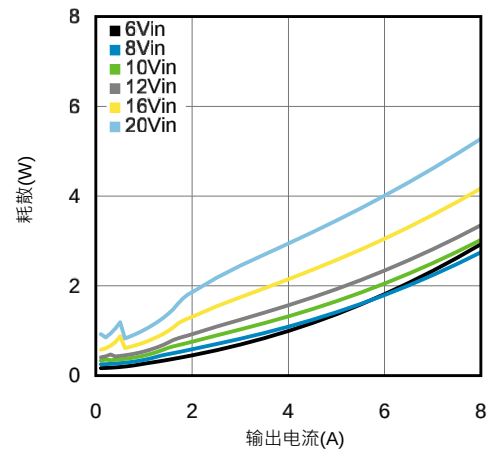
在25°C时3.3V输出耗散
