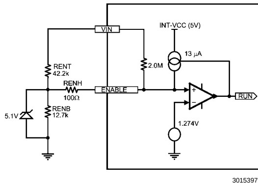
图1. 使能输入详图
