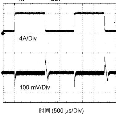
瞬态响应 V_{IN}=12V \cdot V_{OUT}=1.2V 1至8A阶
