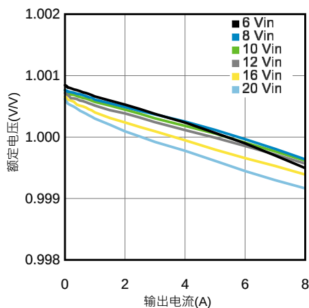
额定线路及负载调节 V_{OUT} = 3.3V
