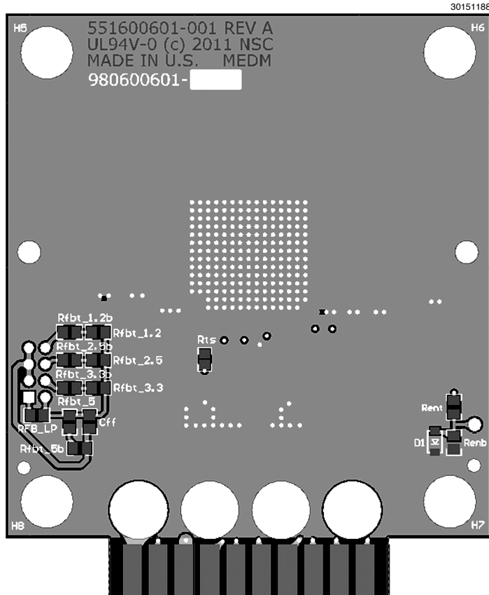
图 6: 布局示例
