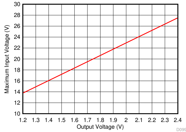
图 9-3. Maximum Input Voltage for V_{OUT} < 2.5 V
