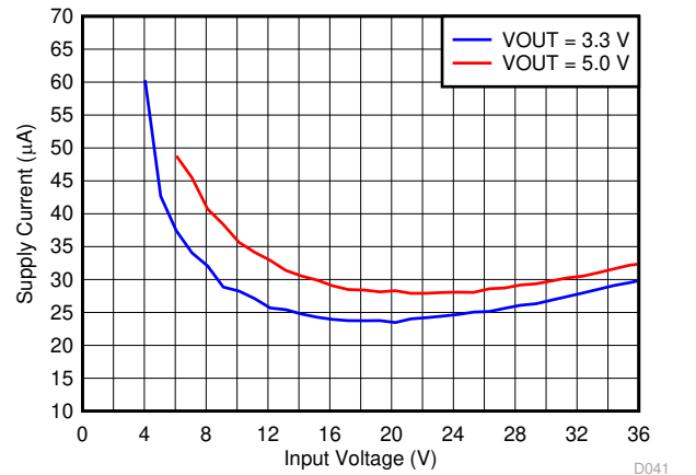
图 7-2. Input Supply Current
