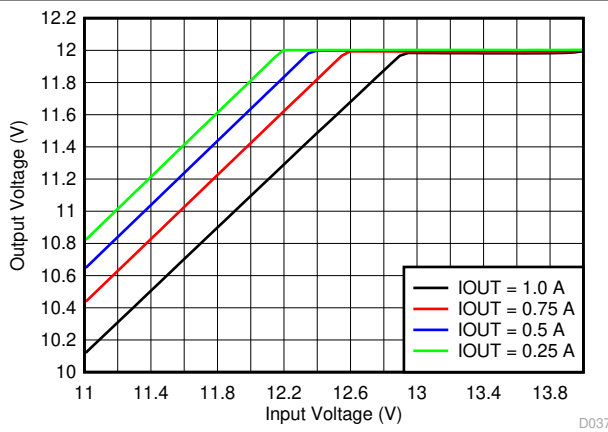
图 6-3. Dropout Voltage
