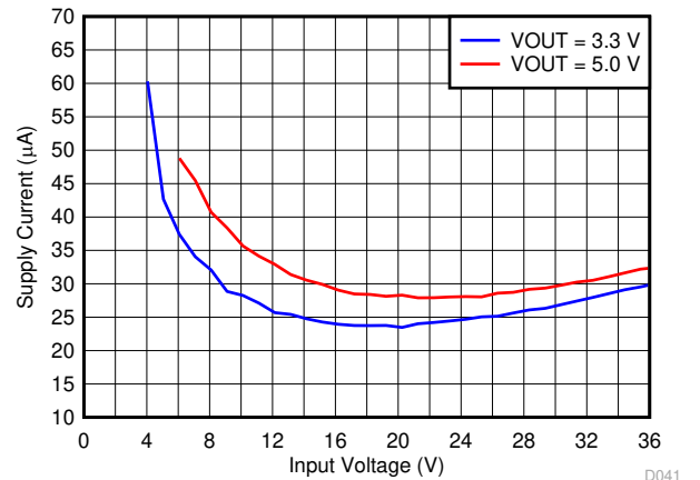
图 6-2. Input Supply Current
