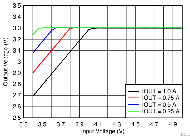
图 6-3. Dropout Voltage
