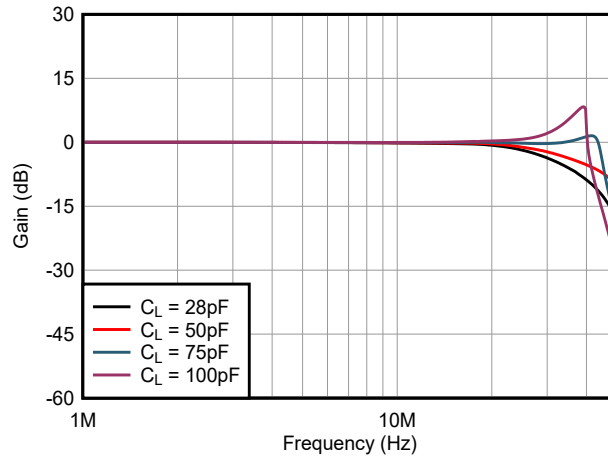
图 5-17. A_4 和 A_5 容性负载响应
