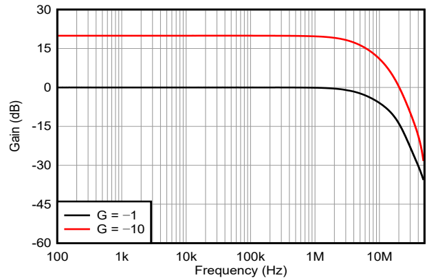
图 5-16. A_4 和 A_5 反相闭环响应
