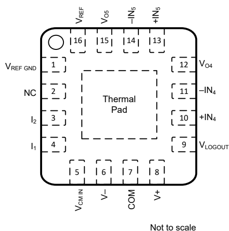
图 4-1. RGV 封装，16 引脚 VQFN ( 俯视图 )
