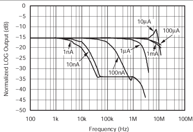
图 5-12. 小信号交流响应 I_2 (10% 正弦调制)
