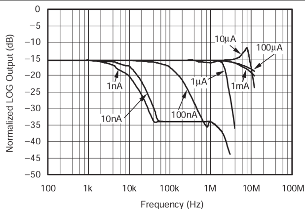
图 5-11. 小信号交流响应 I_1 (10% 正弦调制)
