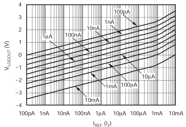
图 5-6. V_{LOGOUT} 与 I_{REF} 间的关系
