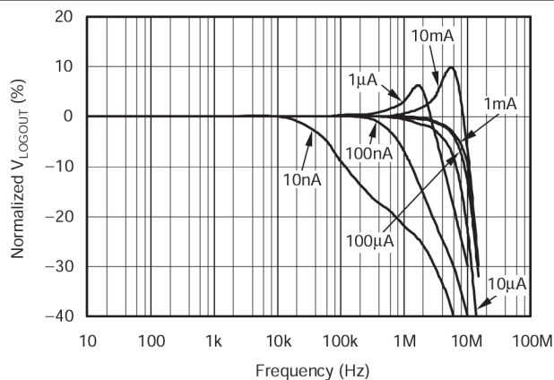
图 5-10. 小信号 V_{LOGOUT}
