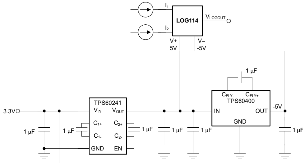
图 7-13. 从 3.3V 电源生成 ±5V 电源
