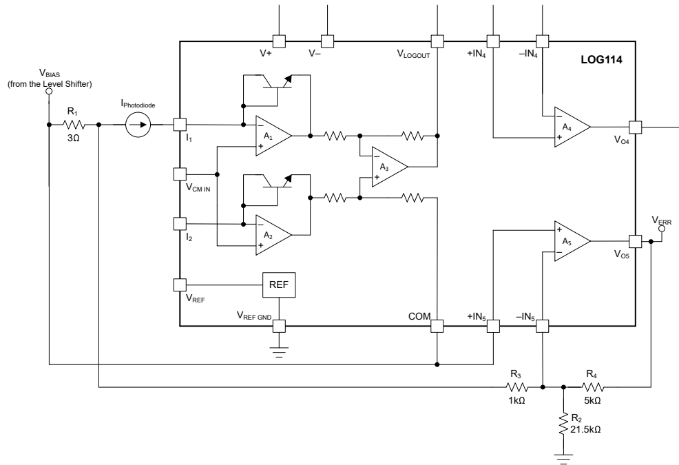
图 7-7. 高电流线性度校正电路
