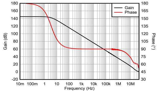
图 5-14. A_4 和 A_5 增益和相位与频率间的关系
