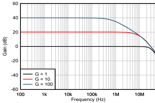
图 5-15. A_4 和 A_5 非反相闭环响应
