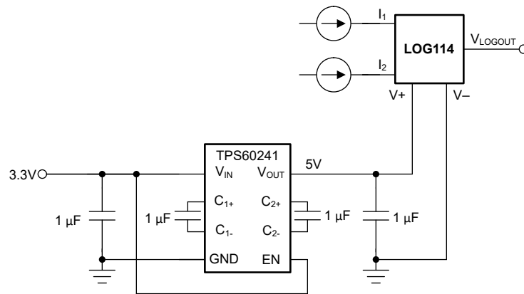
图 7-12. 从 3.3V 电源生成 5V 电源
