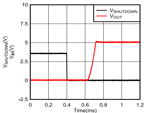
图 5-51. 使能瞬态响应与时间之间的关系 (新芯片)
