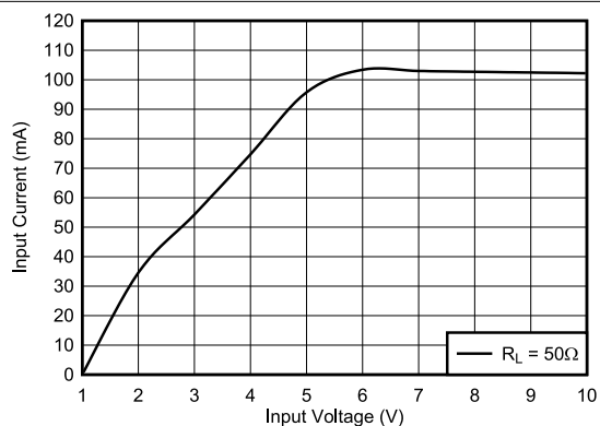
图 5-7. 输入电流与输入电压之间的关系 ( R_L = 50 \Omega ) (旧芯片)
