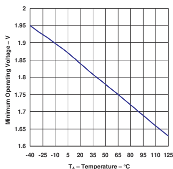
图 5-27. 最低工作电压与温度之间的关系 (旧芯片)
