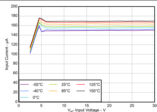
图 5-4. 输入电流与输入电压之间的关系 ( R_L = \text{OPEN} ) (新芯片)
