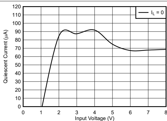
图 5-11. 静态电流与输入电压之间的关系 ( I_L = 0 ) (旧芯片)
