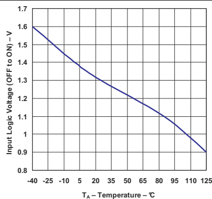
图 5-36. 关断阈值电压 (从关断变为导通) 与温度之间的关系 (旧芯片)
