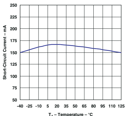
图 5-21. 短路电流与温度之间的关系 (旧芯片)
