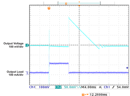
图 5-47. 负载瞬态响应与时间之间的关系 ( V_{OUT} = 5V , C_L = 10\mu F ) (旧芯片)
