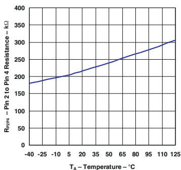
图 5-35. LP2951 分压器电阻与温度之间的关系 (旧芯片)
