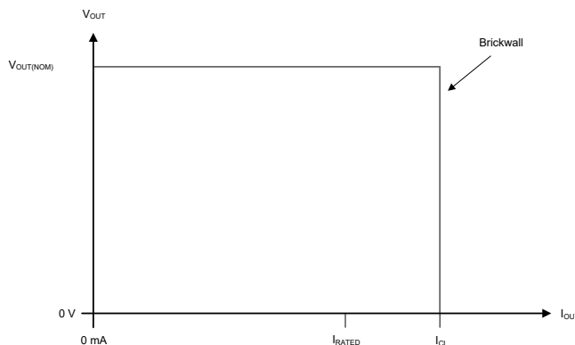
图 6-2. 电流限制
