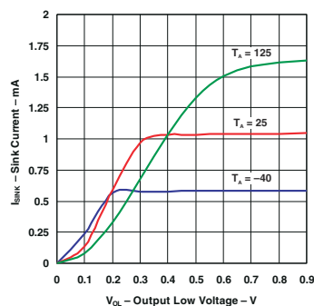
图 5-33. LP2951 \overline{\text{ERROR}} 比较器灌电流与输出低电压之间的关系 (旧芯片)
