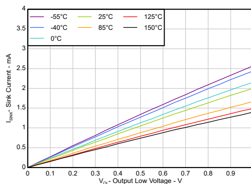
图 5-34. \overline{\text{ERROR}} 比较器灌电流与输出低电压之间的关系 (新芯片)
