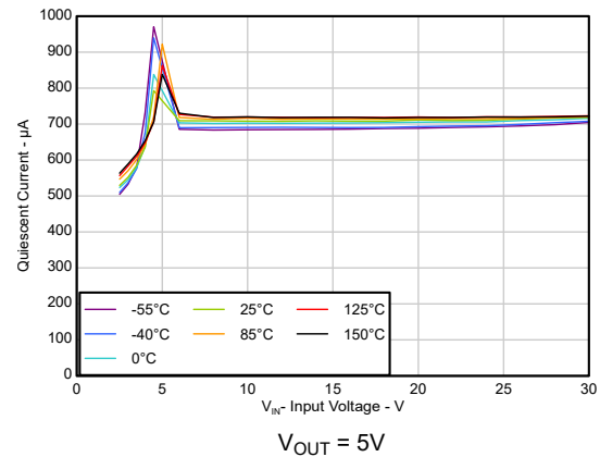
图 5-16. 静态电流与输入电压之间的关系 ( I_L = 100mA ) (新芯片)
