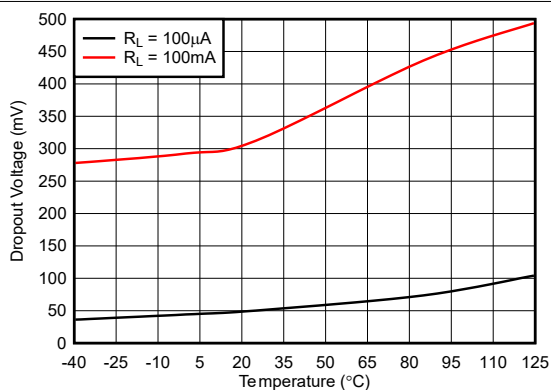
图 5-23. 压降电压与温度之间的关系 (旧芯片)
