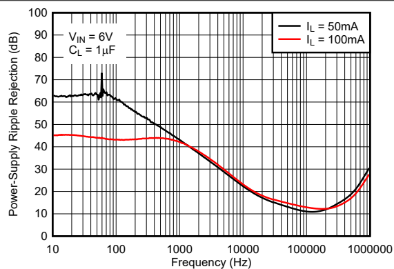
图 5-57. 纹波抑制与频率之间的关系 (旧芯片)
