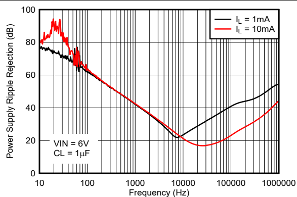
图 5-56. 纹波抑制与频率之间的关系 (旧芯片)
