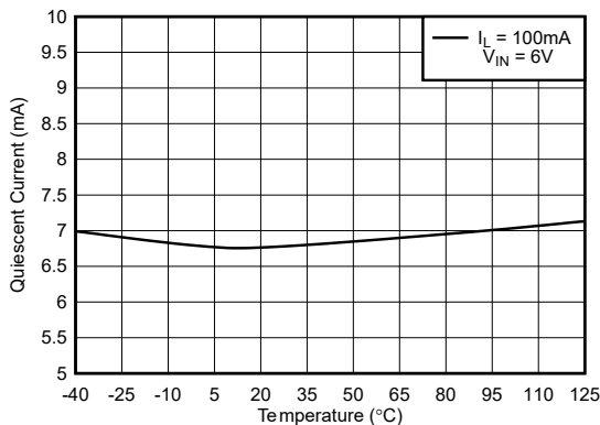
图 5-17. 静态电流与温度之间的关系 ( I_L = 100mA ) (旧芯片)
