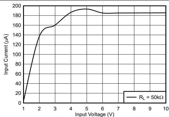
图 5-5. 输入电流与输入电压之间的关系 ( R_L = 50k\Omega )
