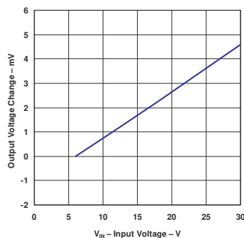
图 5-40. 线性调整率与输入电压之间的关系 (旧芯片)
