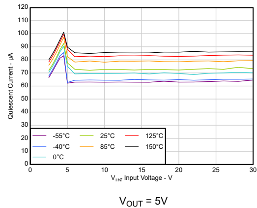
图 5-14. 静态电流与输入电压之间的关系 ( I_L = 1mA ) (新芯片)
