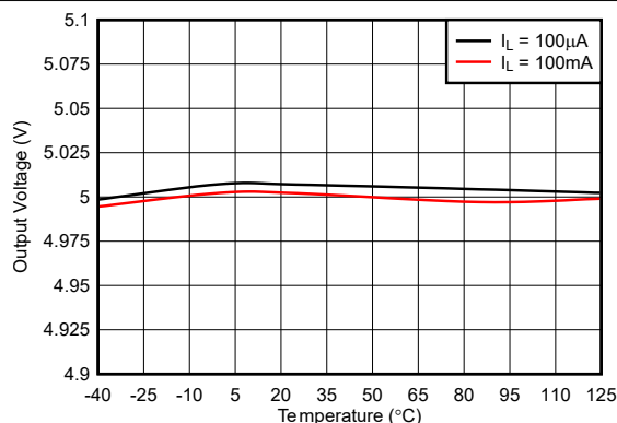
图 5-9. 输出电压与温度之间的关系 (旧芯片)
