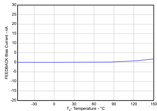
图 5-30. FEEDBACK 偏置电流与温度之间的关系 (新芯片)
