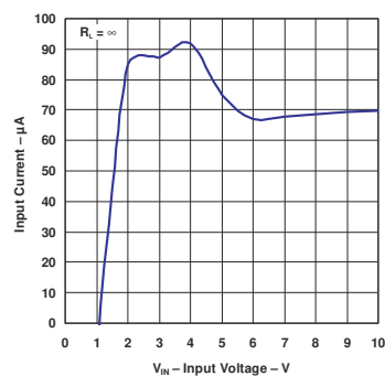
图 5-3. 输入电流与输入电压之间的关系 ( R_L = \text{OPEN} ) (旧芯片)
