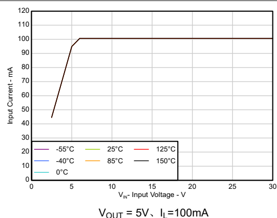
图 5-8. 输入电流与输入电压之间的关系 ( R_L = 50 \Omega ) (新芯片)
