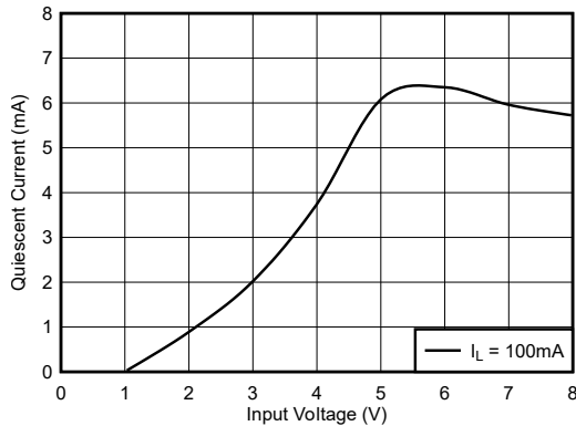
图 5-15. 静态电流与输入电压之间的关系 ( I_L = 100mA ) (旧芯片)
