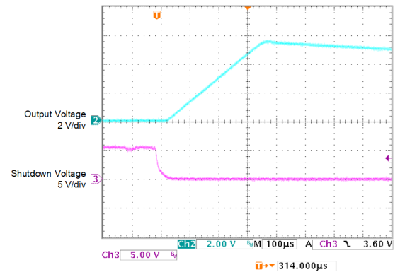
图 5-52. 使能瞬态响应与时间之间的关系 ( I_L = 1mA , C_L = 10 \mu F )
