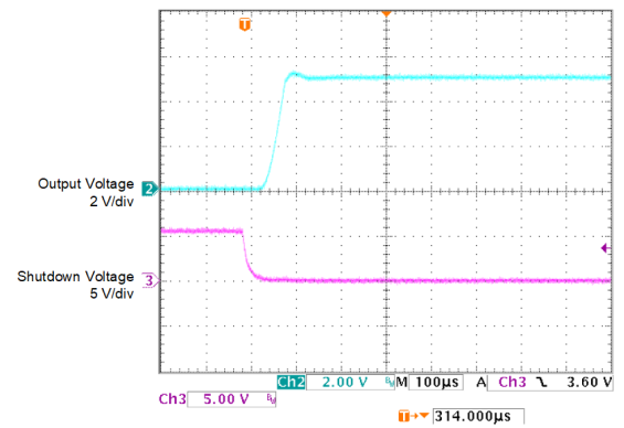
图 5-50. 使能瞬态响应与时间之间的关系 ( I_L = 1mA , C_L = 1 \mu F ) (旧芯片)
