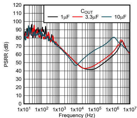
图 5-58. 纹波抑制与频率之间的关系 (新芯片)
