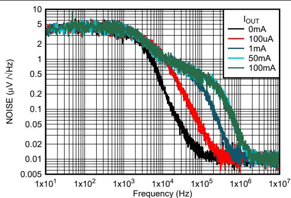
图 5-62. 输出噪声与频率间的关系 (新芯片)
