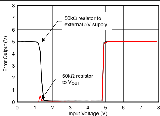
图 5-31. LP2951 \overline{\text{ERROR}} 比较器输出与输入电压之间的关系 (旧芯片)
