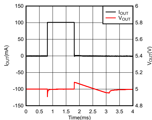
图 7-6. 负载瞬态响应与时间之间的关系 (新芯片)
