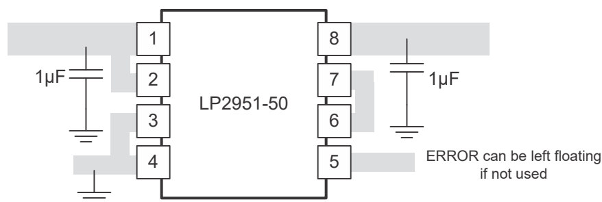
图 7-7. LP2951 布局示例 ( D 或 P 封装 )
