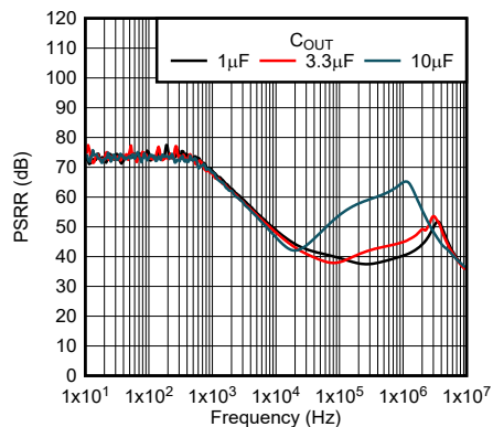
图 5-59. 纹波抑制与频率之间的关系 (新芯片)
