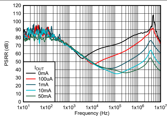
图 5-56. 纹波抑制与频率之间的关系 (旧芯片)
