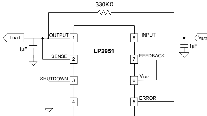
图 7-2. 12V 至 5V 转换器
