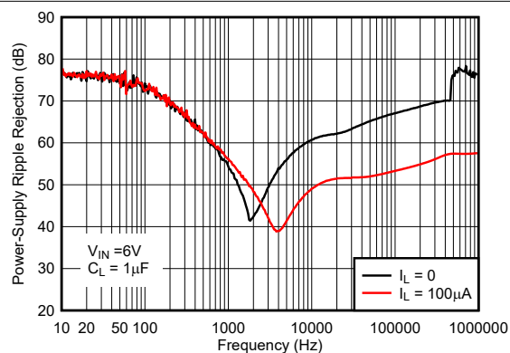
图 5-55. 纹波抑制与频率之间的关系 (旧芯片)
