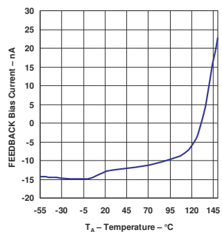
图 5-29. LP2951 FEEDBACK 偏置电流与温度之间的关系 (旧芯片)
