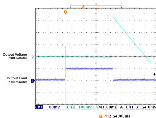
图 7-5. 负载瞬态响应与时间之间的关系 (旧芯片)
