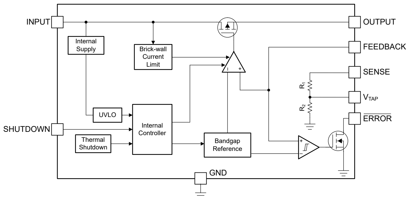
图 6-1. LP2951 功能框图
