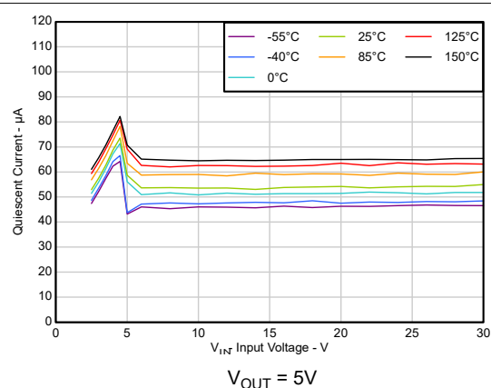
图 5-12. 静态电流与输入电压之间的关系 ( I_L = 0 ) (新芯片)
