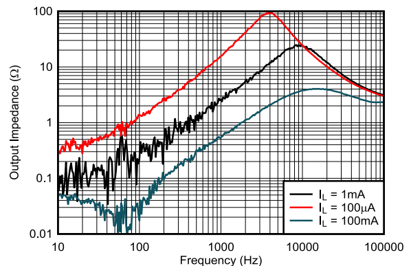
图 5-54. 输出阻抗与频率间的关系 (旧芯片)
