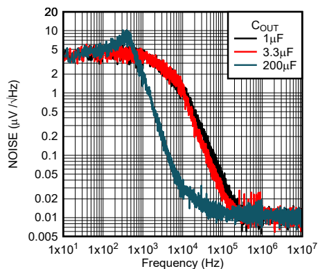
图 5-62. 输出噪声与频率间的关系 (新芯片)
