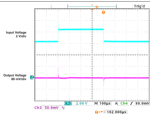
图 5-45. 线路瞬态响应与时间之间的关系 (旧芯片)
