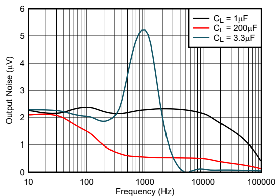
图 5-61. 输出噪声与频率之间的关系 (旧芯片)
