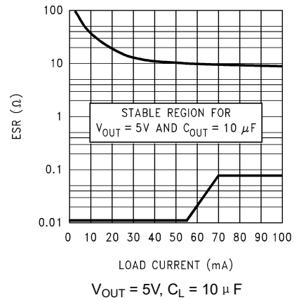
图 7-4. 5V, 10 μ F ESR Curves (Legacy Chip)
