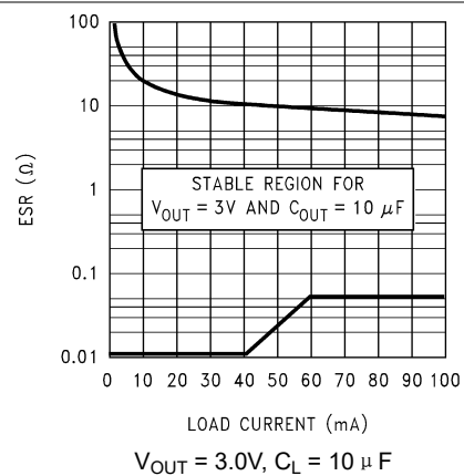
图 7-6. 3.0V, 10 \mu F ESR Curves (Legacy Chip)
