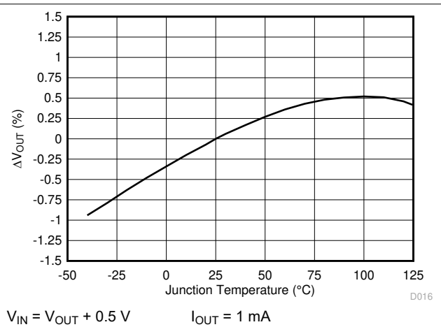
图 6-16. \Delta V_{OUT} vs Temperature
