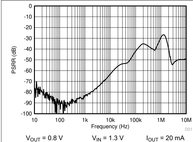
图 6-11. PSRR vs Frequency
