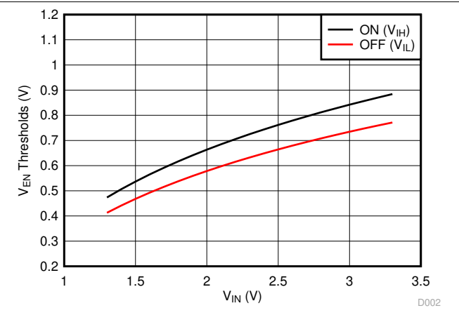
图 6-2. V_{EN} Thresholds vs V_{IN}
