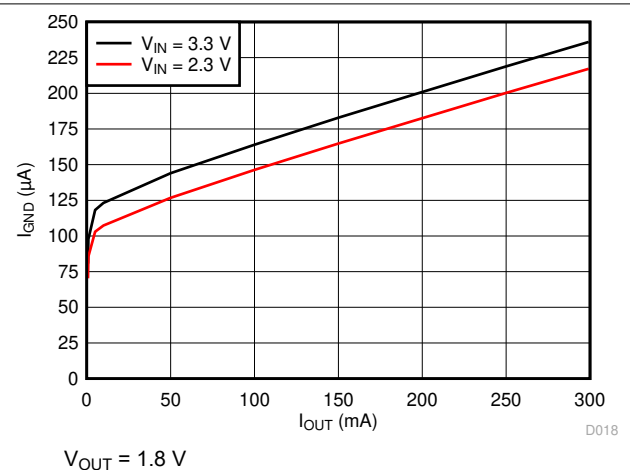
图 6-18. I_{GND} vs I_{OUT}
