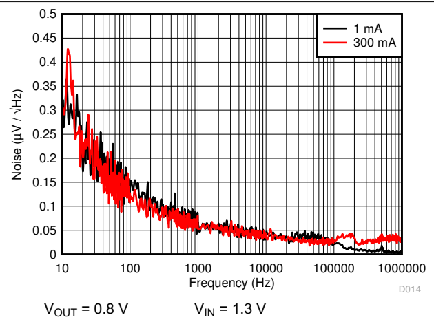
图 6-14. Noise Density
