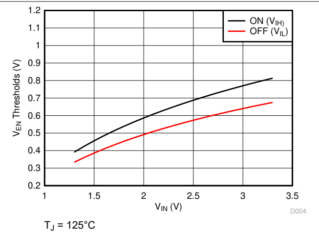
图 6-4. V_{EN} Thresholds vs V_{IN}
