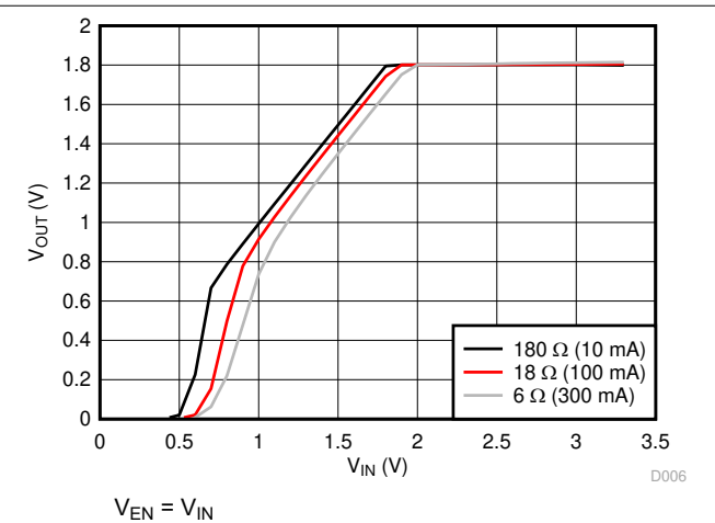
图 6-6. V_{OUT} vs V_{IN}
