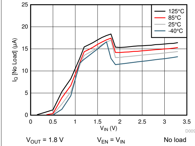
图 6-9. I_Q vs V_{IN}
