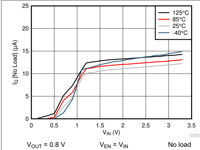
图 6-7. I_Q vs V_{IN}
