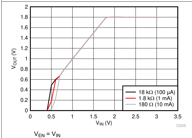
图 6-5. V_{OUT} vs V_{IN}
