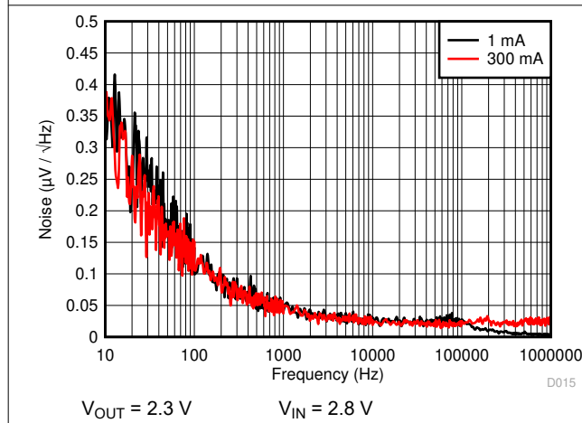
图 6-15. Noise Density
