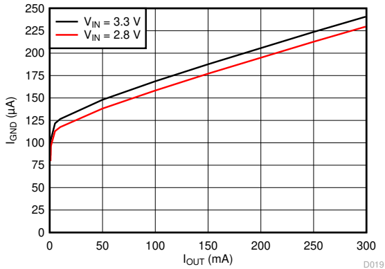
图 6-19. I_{GND} vs I_{OUT}
