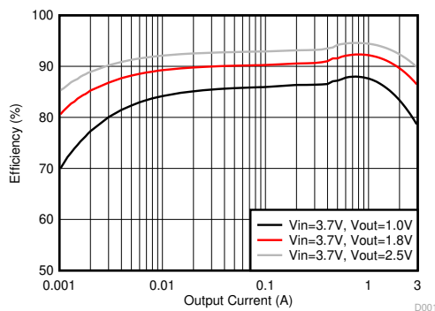
直流/直流效率与输出电流间的关系
