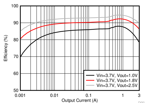
直流/直流效率与输出电流间的关系
